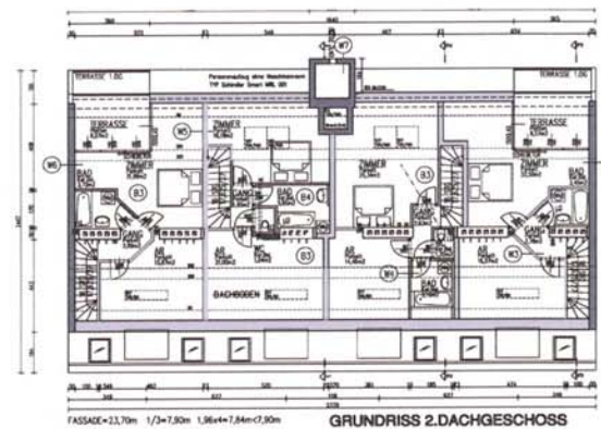
GRUNDRISS 2. DACHGESCHOß
