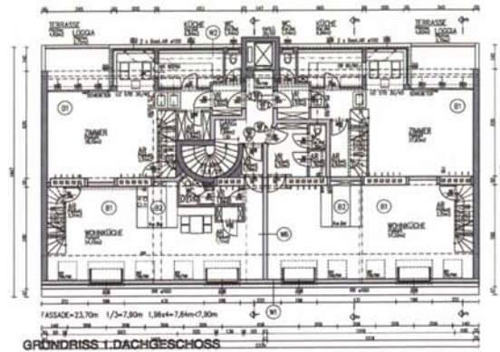
GRUNDRISS 1. DACHGESCHOß
